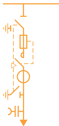
Ячейка контактора и плавких предохранителей CRM (750 мм)
