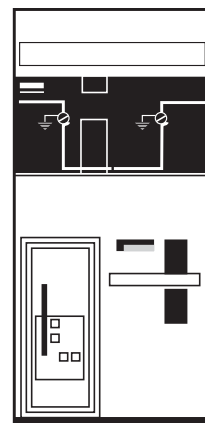
Ячейка выключателя с двумя разъединителями и отходящей линией направо или налево DM2 (750 мм)
