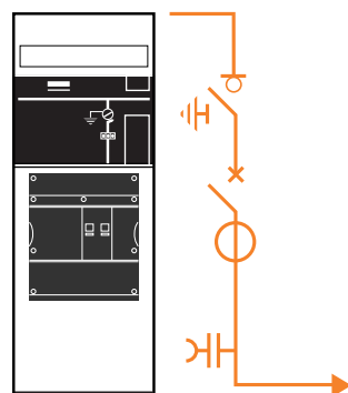
Ячейка с вакуумным выключателем с шинным отводом направо DMV-D (625 мм)
